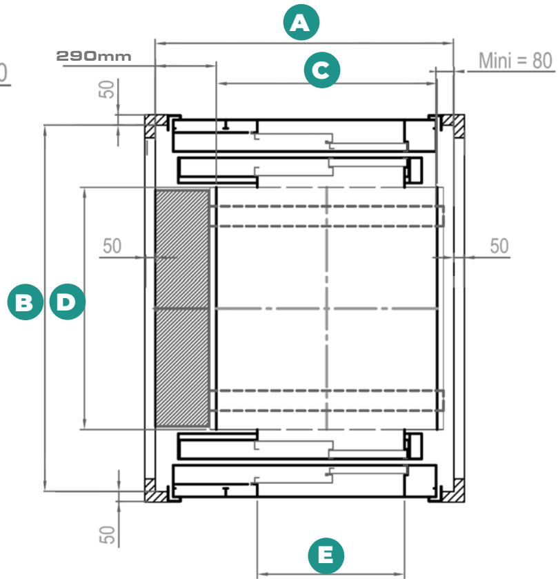
Pylône Pylon
