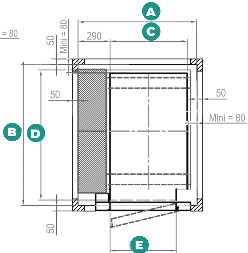
Pylône Pylon
