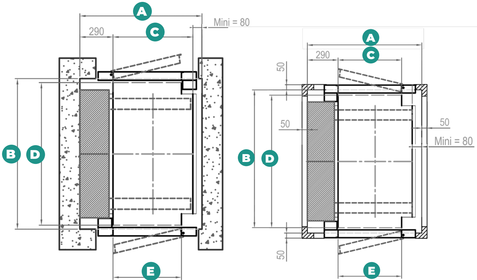
Pylône Pylon
